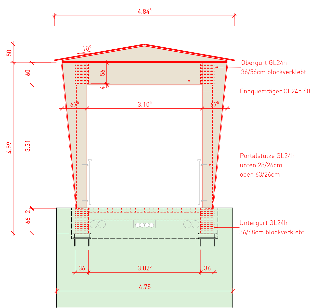
Ansicht Portal 1:50
