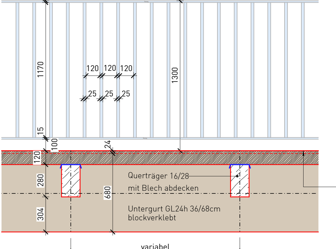
Detail 4 Geländer 1:20
