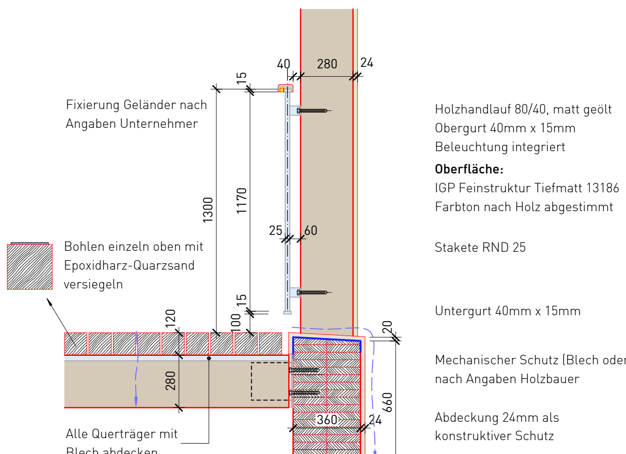
Detail 5 Geländer 1:20
