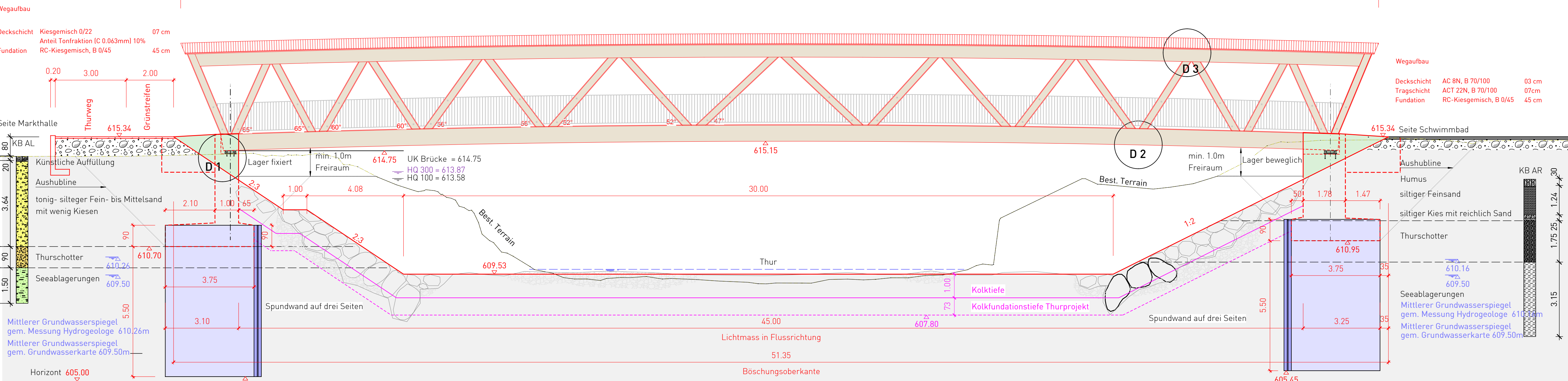
Ansicht A 1:100
