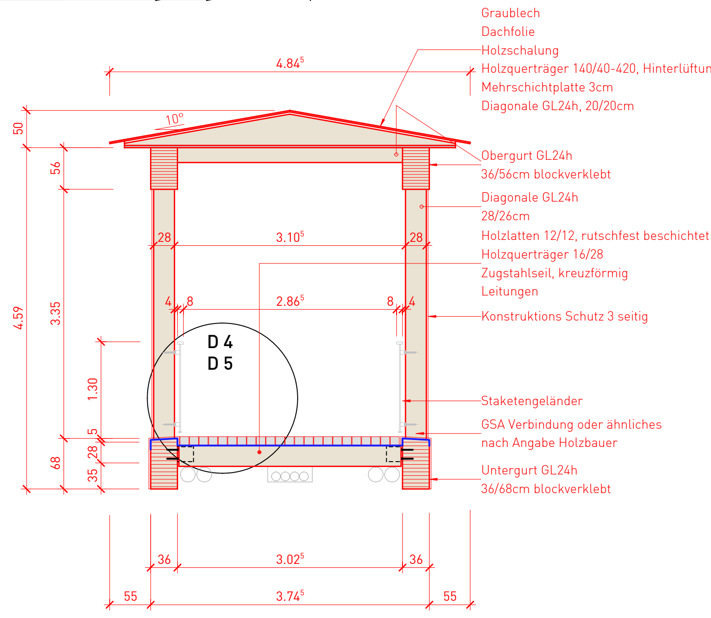
Querschnitt 1:50
